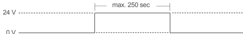
Abb. 4 - Schematische Darstellung Spannungsfreischtaltung
